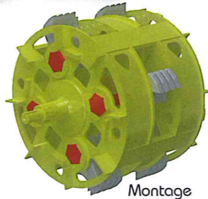
Montage avec 24 fléaux mobiles
