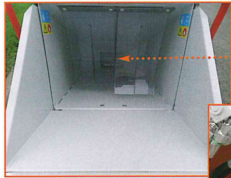
Montage avec 6 outils coupants fixes
